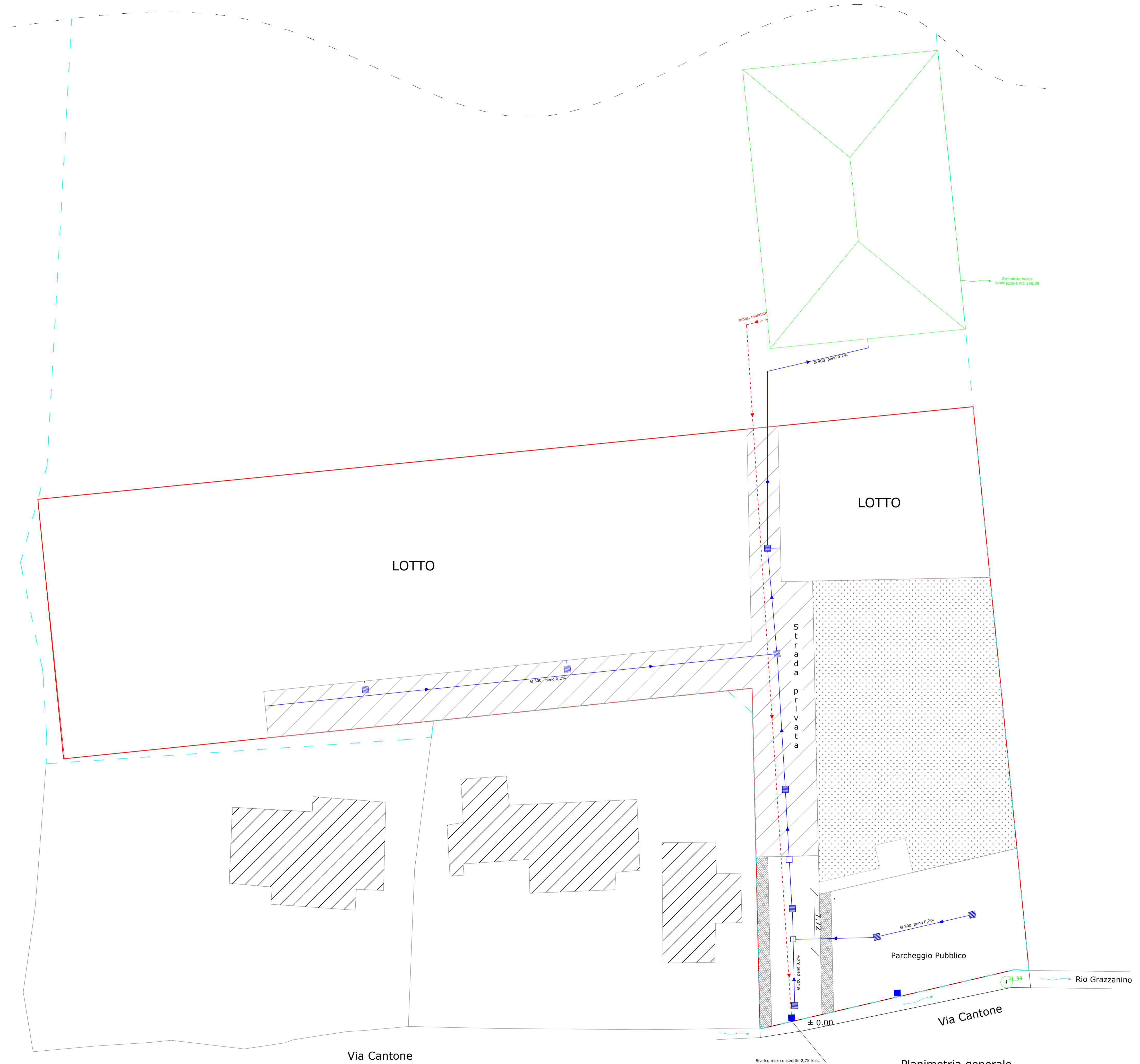
Planimetria generale scala 1:250
